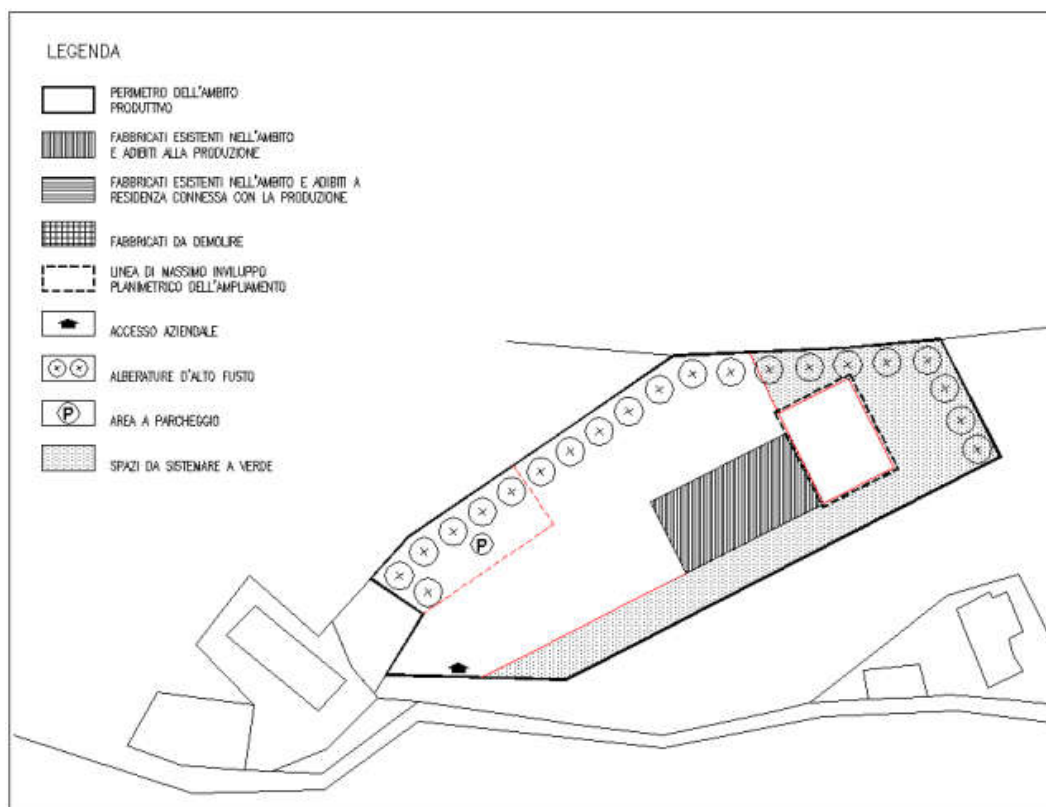
SCHEMA PLANIMETRICO DI PROGETTO 1:500
